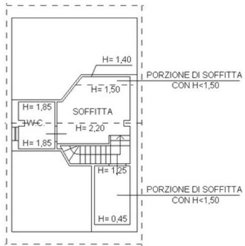
PIANO SECONDO
